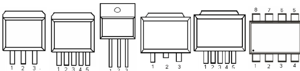
1)TO263-3L 2)TO263-5L 3)TO220-3L 4)TO252-3L 5)TO252-5L 6)SOP8L-EP
