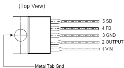
(1) TO220-5L
