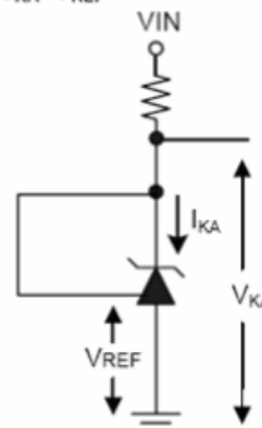
Fig1: V_{KA} = V_{REF}
