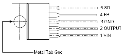
(1) TO220-5L
