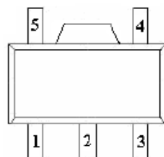
SOT89-5L
