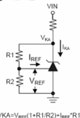
Fig2: V_{KA} > V_{REF}
