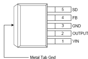
(3) TO263-5L
